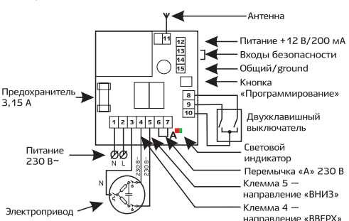
Рис. 1 — Подключение Radio 8113 IP65
