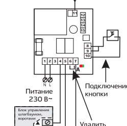
Рис. 3 — Подключение к раздельным входам «ОТКРЫТЬ» и «ЗАКРЫТЬ»
