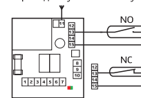
Рис. 4 — Подключение геркона
